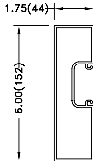
JAMB-6"
