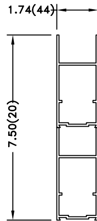
8" NOMINAL MUNTIN BAR
