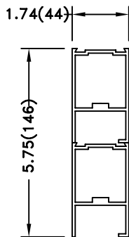
6" NOMINAL MUNTIN BAR
