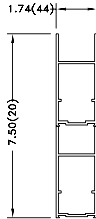
8" NOMINAL MUNTIN BAR
