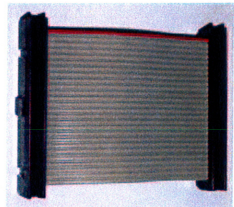
EAU.0006 TCP51 / TCP101 Flat Cable
